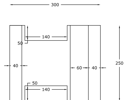
SEZIONE A-A
